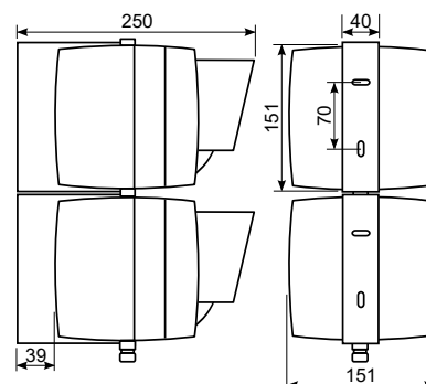
Doppelleuchte mit Verschraubung kombinierbar
